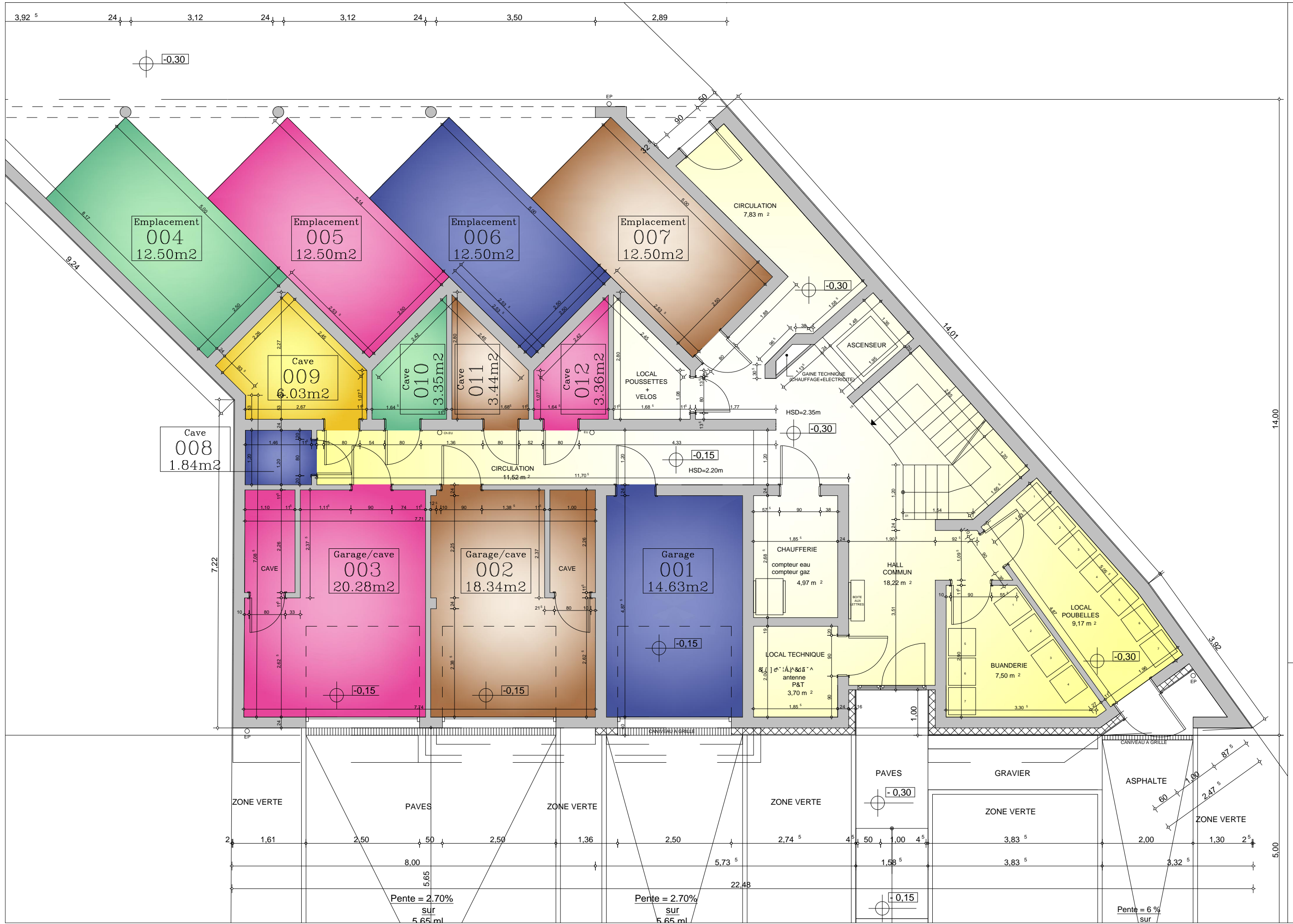
VUE EN PLAN REZ-DE-CHAUSSEE Residence "ANDY" 34, rue de Noertzange KAYL
