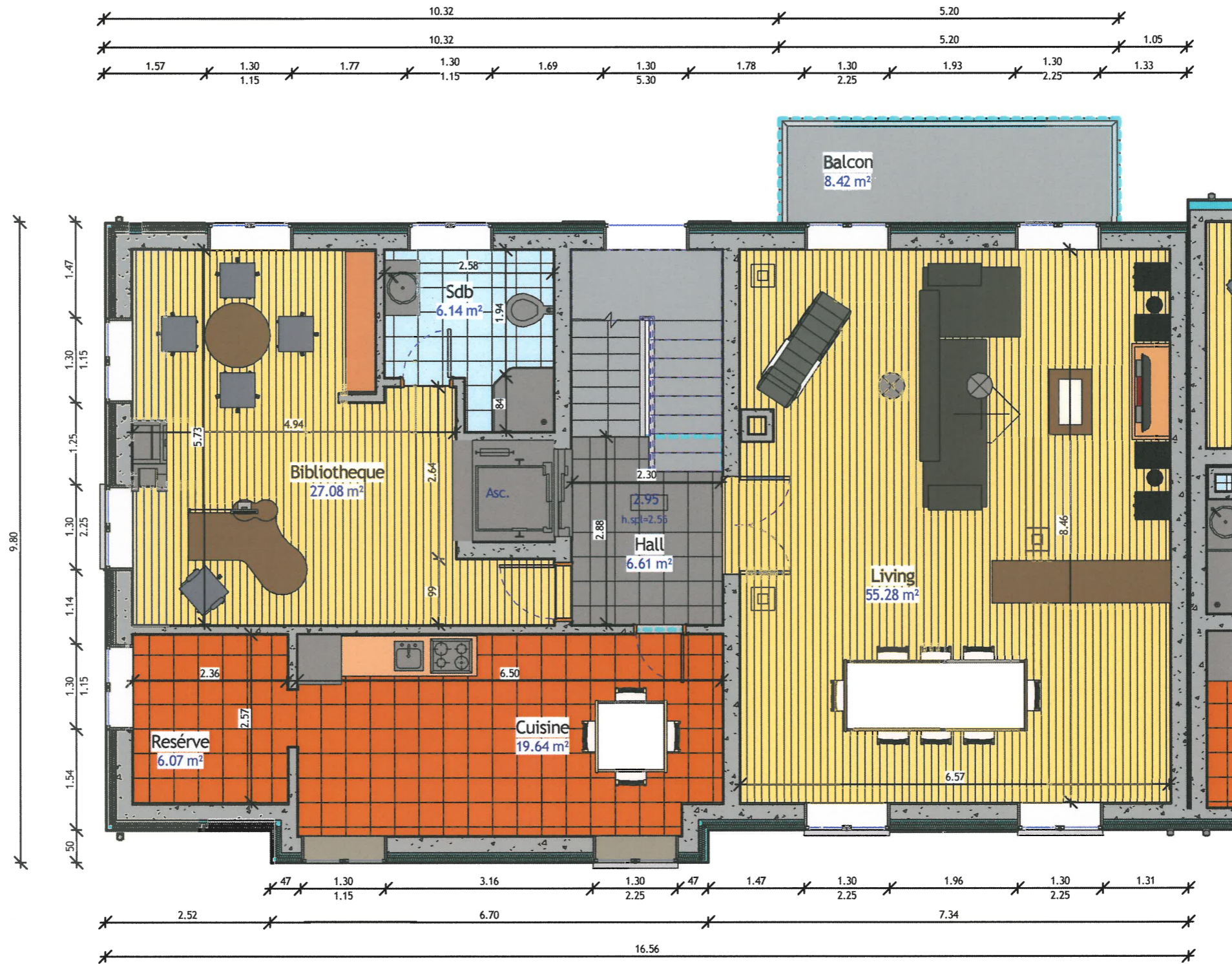
1 maison n. ° 1_première étage Ech : 1 : 75
